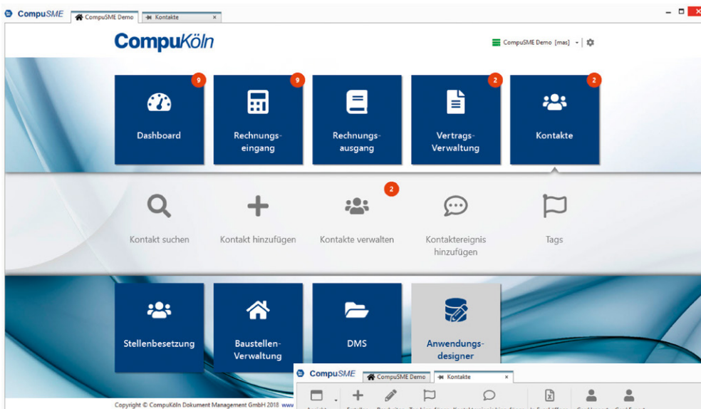
CompuDMS-Hauptansicht
