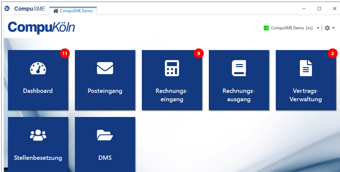
CompuSME-Hauptansicht
