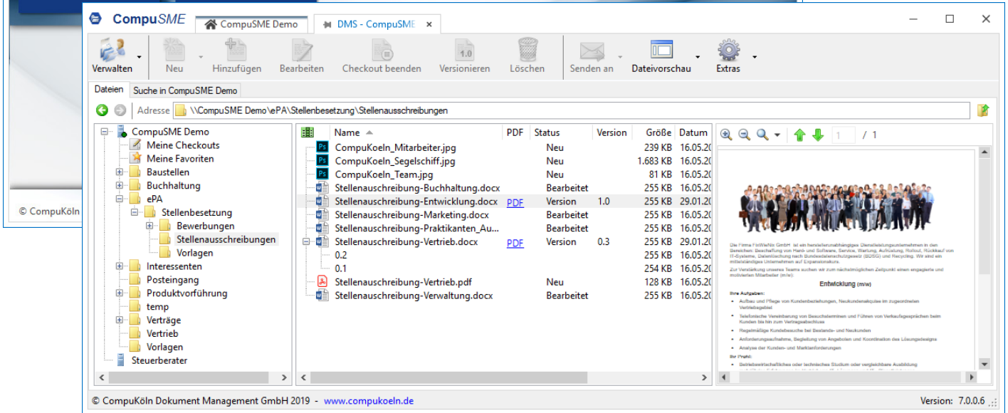
Dokumentenverwaltung
